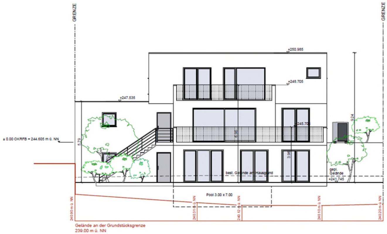
Ansicht Süd
