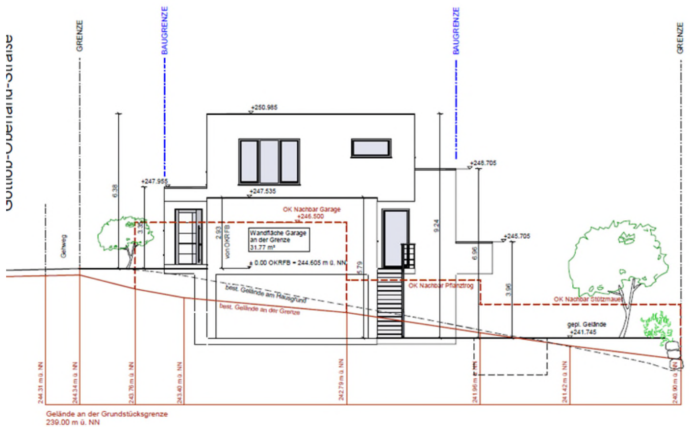
Ansicht West
